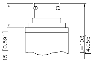
E - 4 pole connector EN 175301-803 type A
