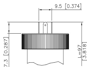
M - 4 pole connector EN 175301-803 type C
