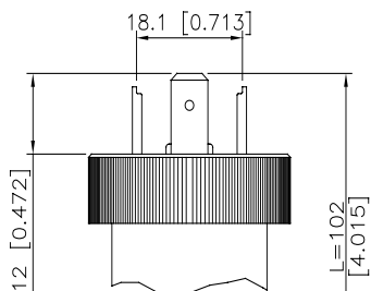
E - 4 pole connector EN 175301-803 type A
